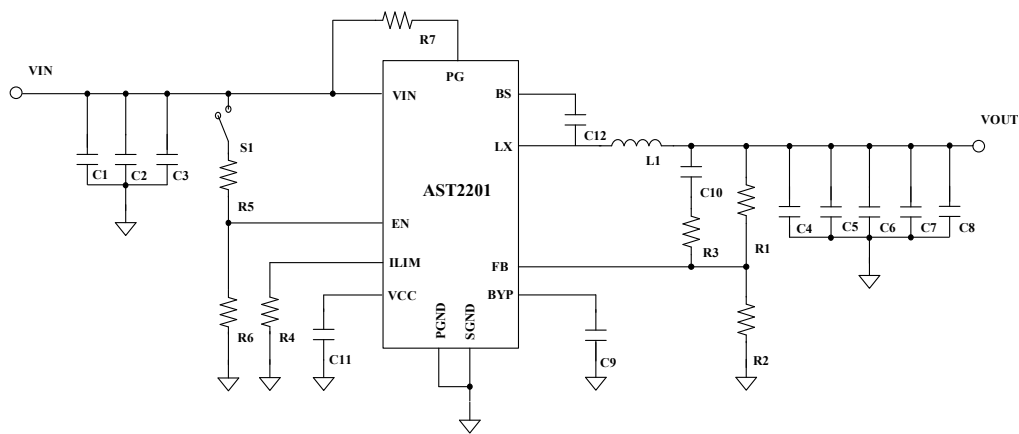
图 3 AST2201 应用图
