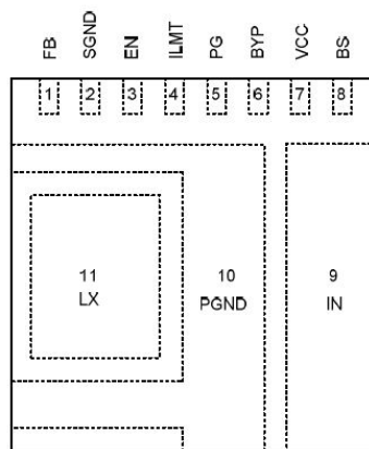
图 1 引脚分布图(顶视图)
