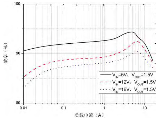
图 2 效率曲线
