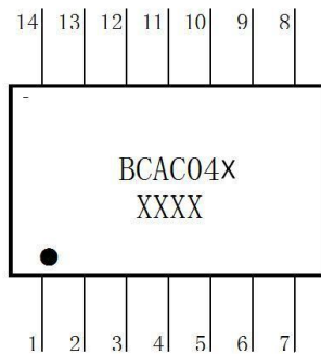
图 2 器件打印标志示意图
